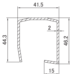
1710 Армирование 44.3 * 41.5 * 46.0 * 2.0 мм
