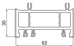
3297 Расширитель 30 мм
