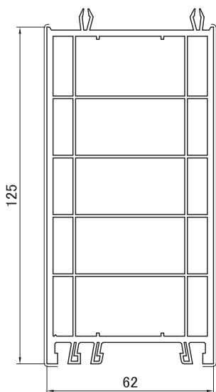
3293 Расширитель 125 мм
