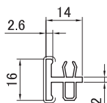
1247 Межрамный соединительный профиль
