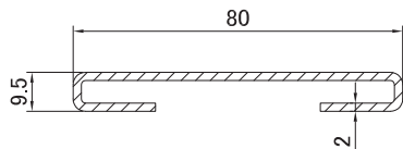
1712 Армирование 9.5 * 80.0 * 2.0 мм
