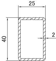
3716 Армирование 40.0 * 25.0 мм
