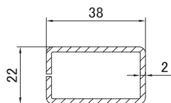
1720 Армирование 22.0 * 38.0 мм
