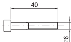
3462 ☉ Винт М6 * 40
