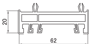
3298 Расширитель 20 мм
