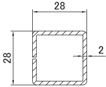
1701 Армирование 28.0 * 28.0 мм
