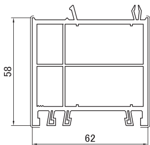
3289 Расширитель 58 мм
