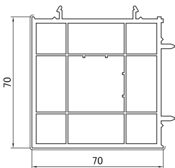
1243 Соединительный профиль 90°
