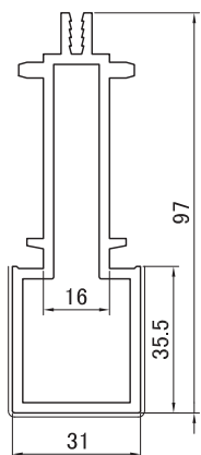
3291 Статический соединительный профиль
