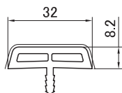
3292 Закрывающий профиль для 3291
