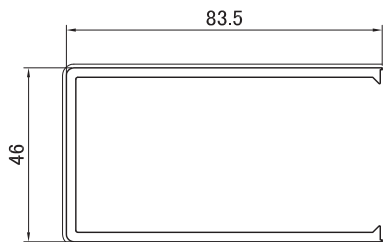
3240 Декоративный закрывающий профиль для пилястра
