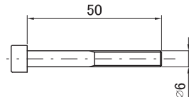
3464 ☉ Винт М6 * 50
